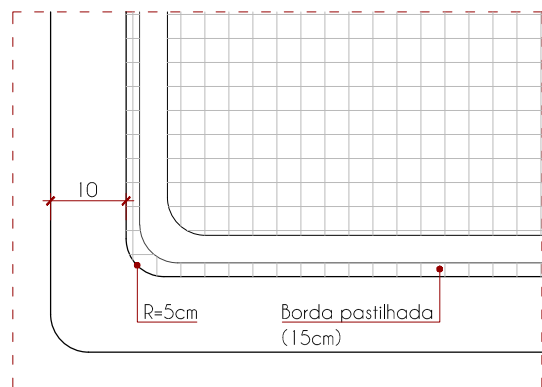
Ampliação borda 1/10
