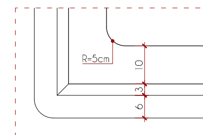
Ampliação borda 1/10
