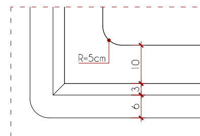
Ampliação borda 1/10
